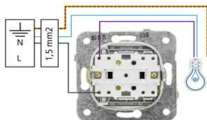
Va et vient - Simple allumage
