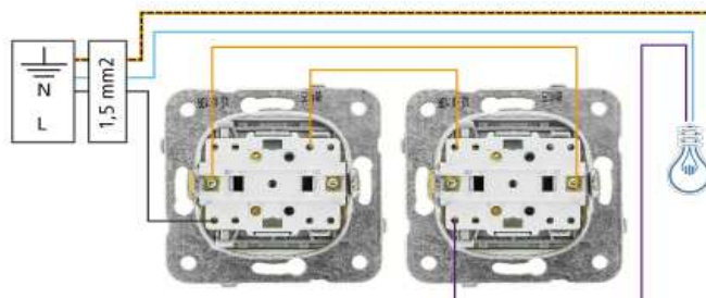
Va et vient - 2 points d'allumages
